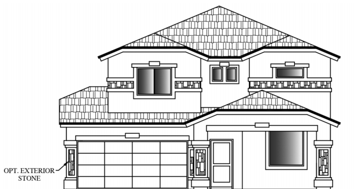
ELEVATION B
