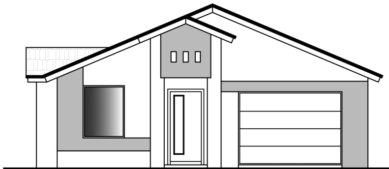
ELEVATION A
