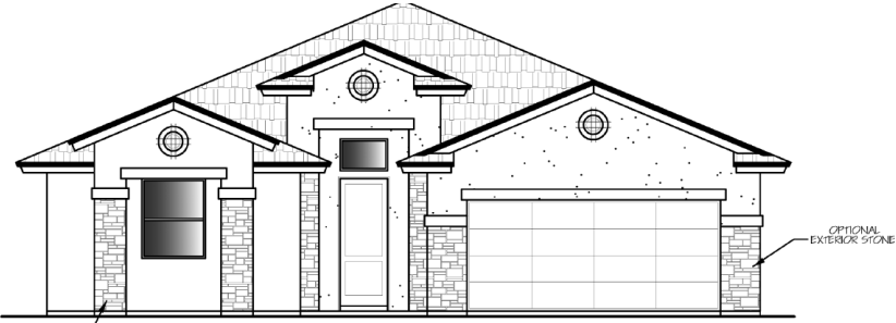
ELEVATION B
