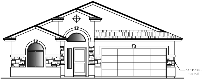
ELEVATION B
