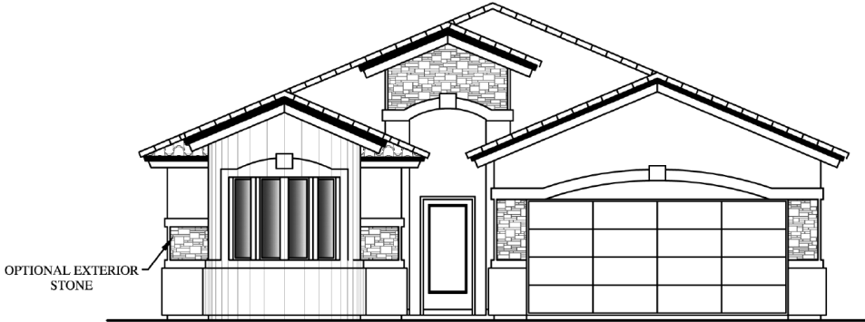
ELEVATION B
