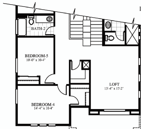
BEDROOM 5
