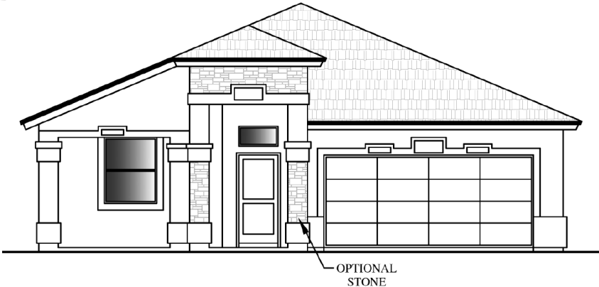
ELEVATION B
