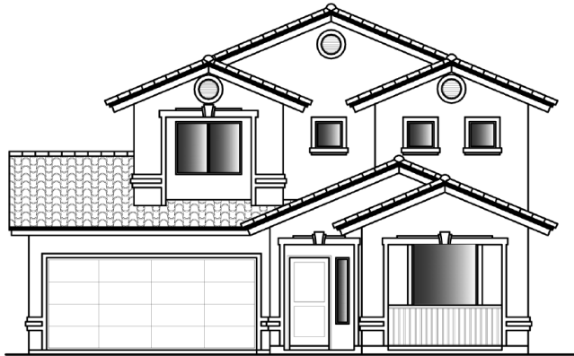
ELEVATION A
